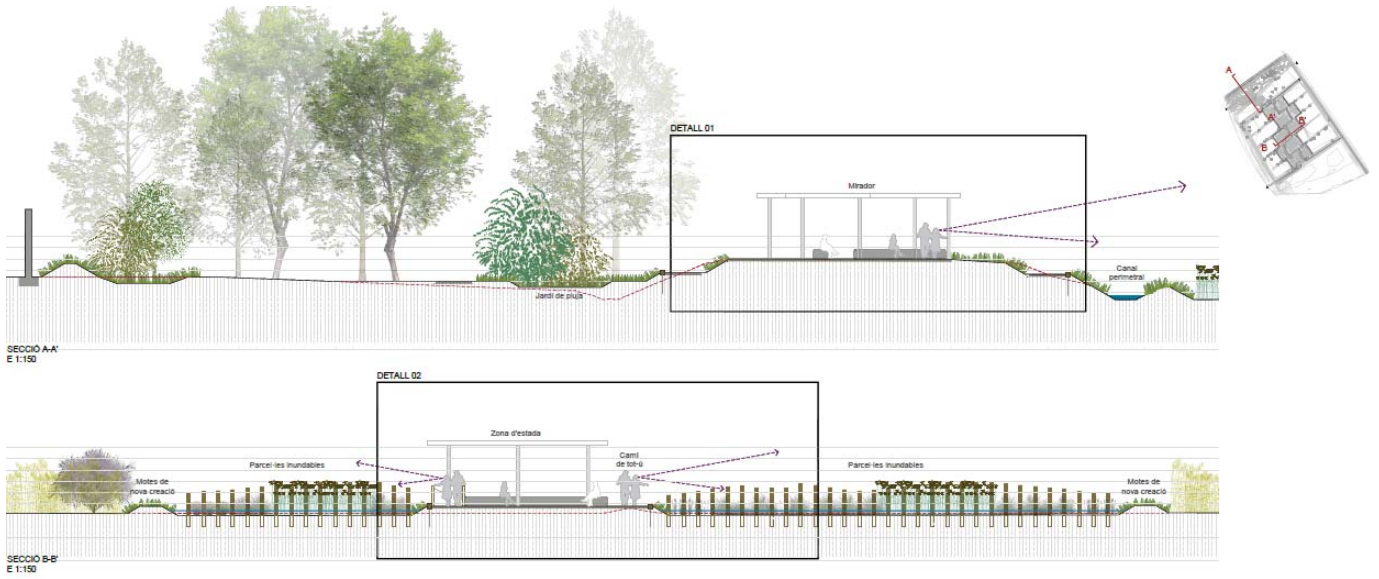
Figura 7 Seccions tipus - Detalls executius
