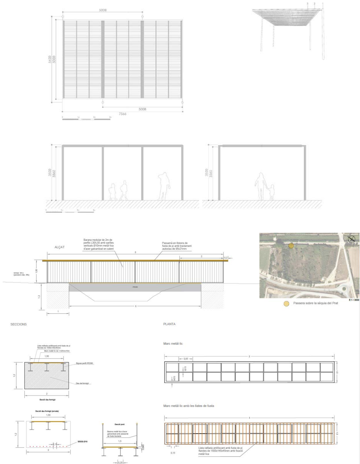
Figura 9 Detall de les estructures d'ús social
