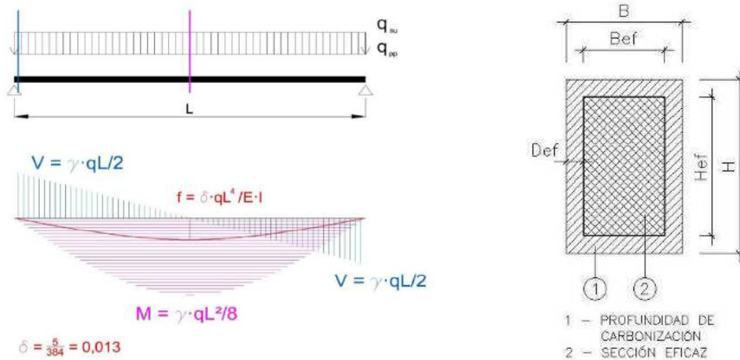
Ley de esfuerzos en una de las vigas de la pasarela y sección tipo de la viga
