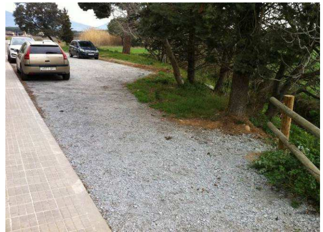
Sistema de cunetes i trenques per derivar l'aigua al torrent
